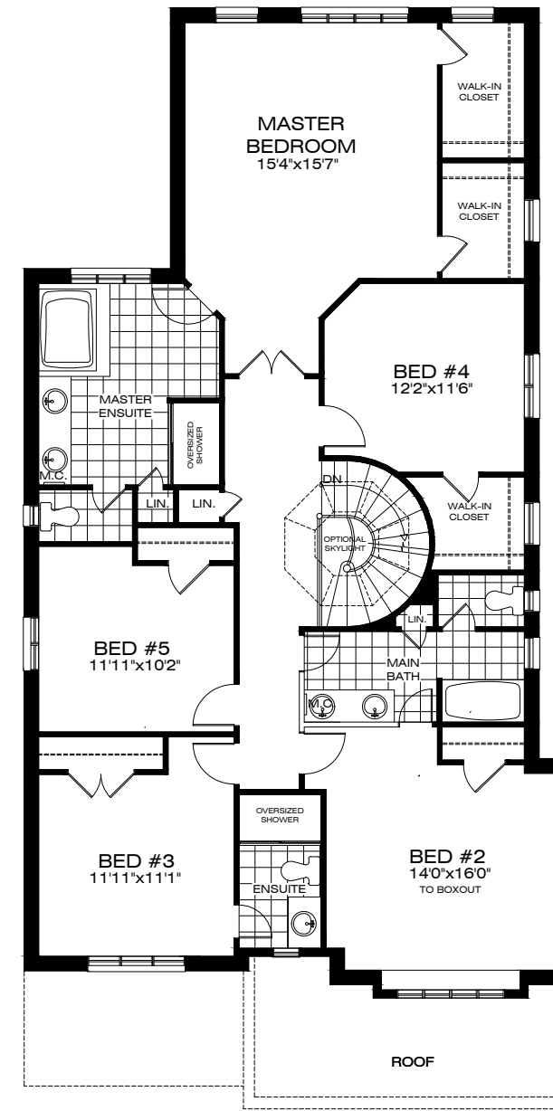
OPTIONAL 5 BEDROOM PLAN 'A'
